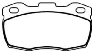
PFC380001 Dimensões em MM: 153,30 x 63,50 x 14,50
