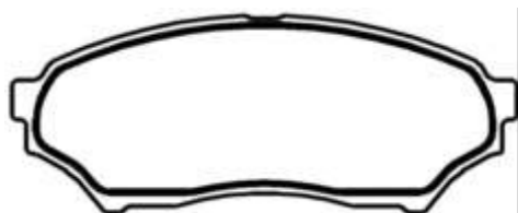
PFC390004 Dimensões em MM: 123,30 x 48,10 x 15,30
