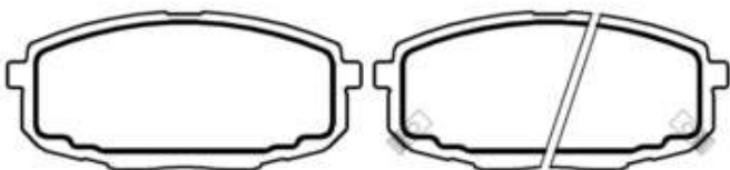
PFC320009 Dimensões em MM: 153,81 x 58,28 x 17,50
