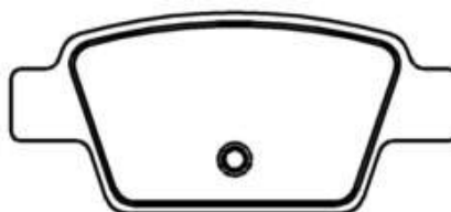
PFC030020 Dimensões em MM: 136,80 x 57,00 x 19,00
