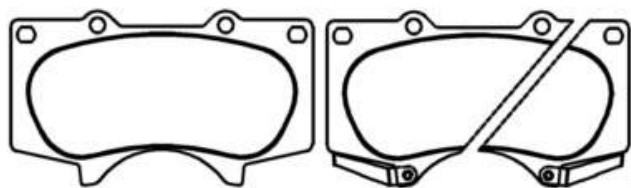
PFC220007 Dimensões em MM: 119,00 x 68,00 x 17,00
