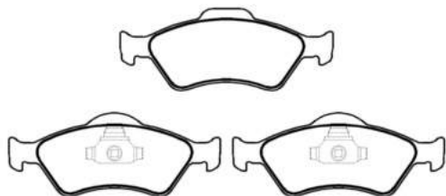
PFC100008 Dimensões em MM: 117,94 x 61,11 x 15,50
