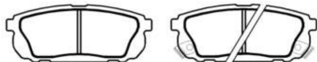
PFC330009 Dimensões em MM: 155,00 x 60,00 x 17,00
