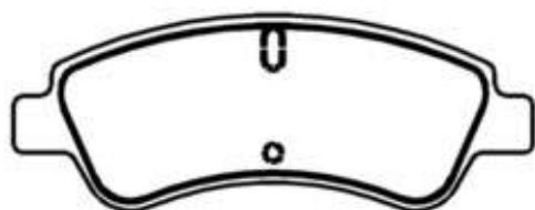
PFC170002 Dimensões em MM: 129,60 x 55,86 x 18,30
