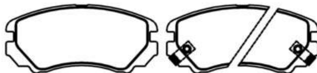
PFC320011 Dimensões em MM: 129,20 x 72,75 x 18,00
