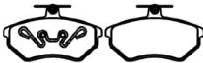
PFC010022 Dimensões em MM: 156,20 x 74,00 x 19,50
