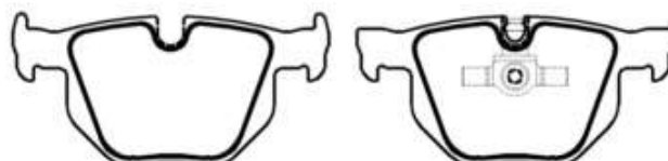
PFC260001 Dimensões em MM: 146,85 x 59,60 x 17,50
