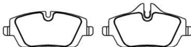
PFC240002 Dimensões em MM: 150,00 x 57,50 x 17,50
