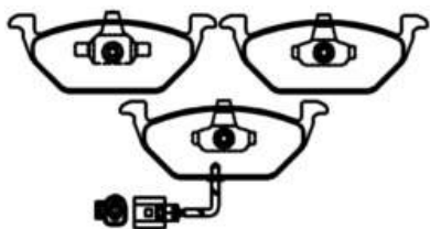
PFC010016 Dimensões em MM: 146,00 x 54,70 x 19,00
