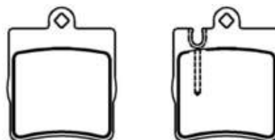
PFC020014 Dimensões em MM: 173,50 x 85,00 x 27,00 Dimensões em MM: 185,50 x 85,00 x 34,00
