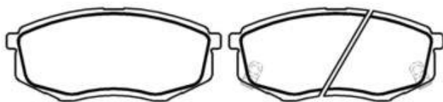
PFC320006 Dimensões em MM: 93,00 x 41,00 x 14,50
