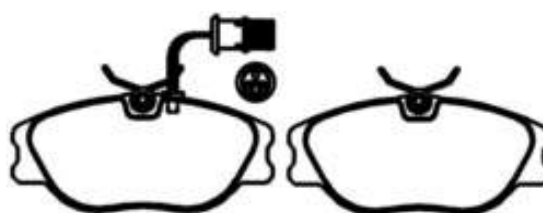
PFC030034 Dimensões em MM: 129,30 x 58,41 x 18,50
