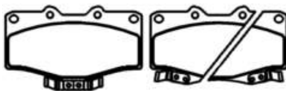
PFC220013 Dimensões em MM: 145,40 x 61,10 x 18,00
