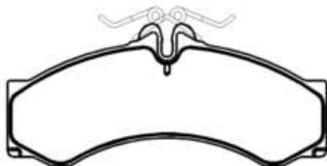
PFC020009 Dimensões em MM: 164,80 x 73,10 x 20,00
