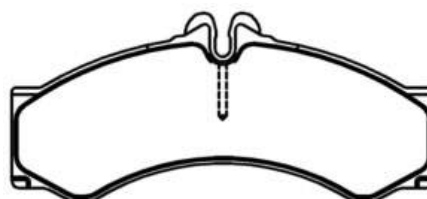
PFC020017 Dimensões em MM: 164,80 x 73,10 x 20,00
