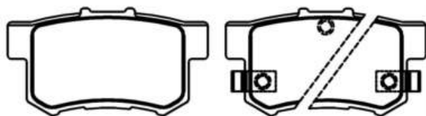
PFC100005 Dimensões em MM: 131,50 x 54,50 x 15,50
