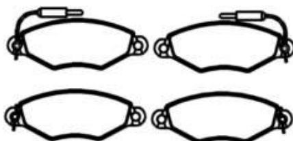
PFC170010 Dimensões em MM: 130,92 x 47,21 x 17,80
