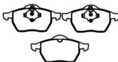
PFC010025 Dimensões em MM: 156,20 x 74,00 x 19,50
