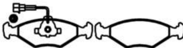
PFC030019 Dimensões em MM: 94,80 x 42,50 x 15,00
