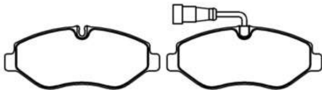
PFC120002 Dimensões em MM: 174,00 x 69,18 x 20,00
