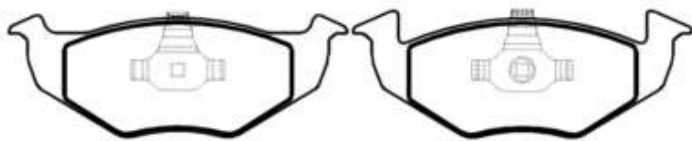
PFC010014 Dimensões em MM: 146,00 x 54,70 x 19,00
