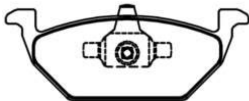
PFC010017 Dimensões em MM: 137,50 x 50,52 x 19,50 Dimensões em MM: 137,50 x 48,31 x 19,50
