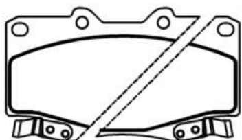
PFC220008 Dimensões em MM: 123,00 x 60,40 x 17,50
