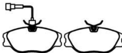
PFC030035 Dimensões em MM: 129,30 x 58,41 x 18,50
