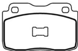
PFC030014 Dimensões em MM: 87,17 x 66,83 x 16,50
