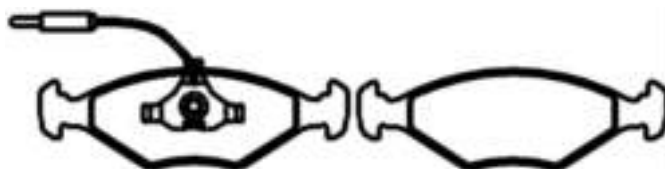
PFC170004 Dimensões em MM: 78,00 x 64,20 x 17,00
