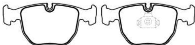
PFC240008 Dimensões em MM: 193,20 x 79,40 x 20,50
